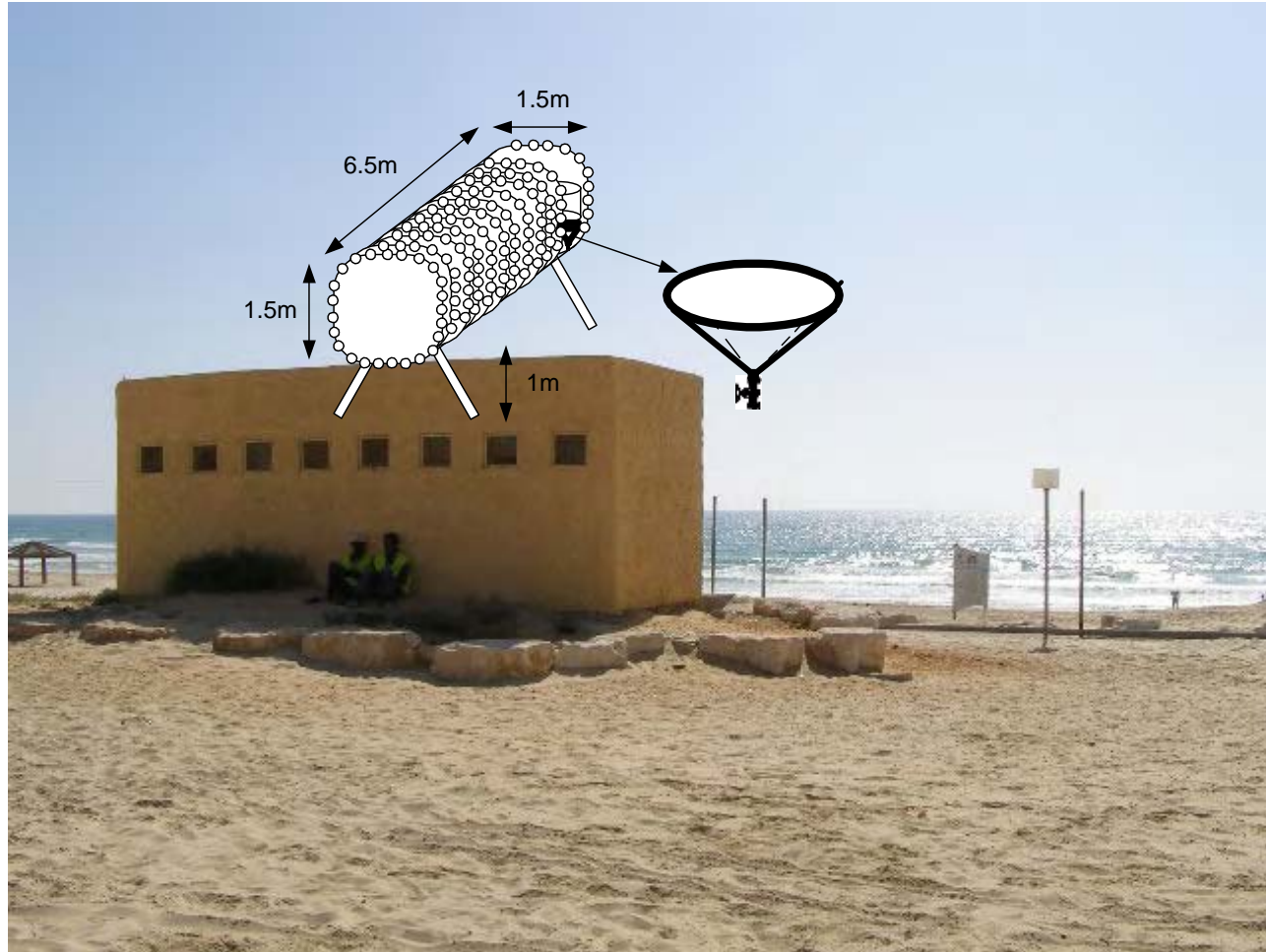
כונס רוח המוצב מעל שירותים ציבוריים על שפת הים, ומייצר 4 קוב מים ביום אשר ישמשו להדחת האסלות
