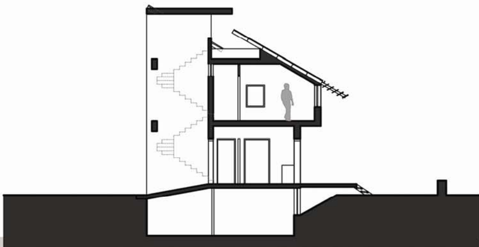
τομή α - α
